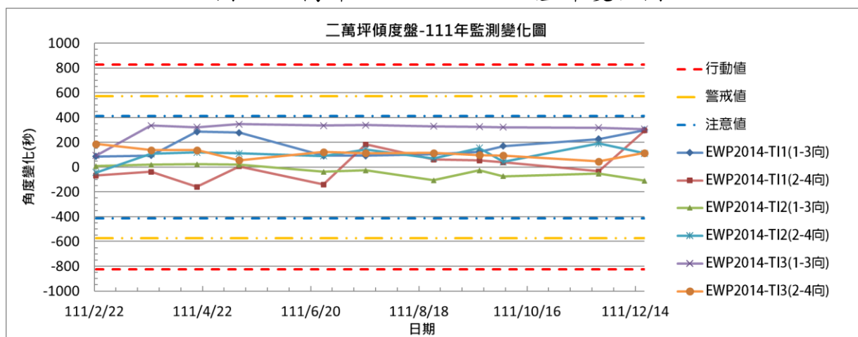
圖 3 二萬坪傾度盤歷時變化圖
