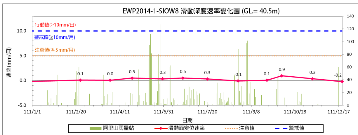
圖 1 二萬坪 EWP2014-1-SIOW8 歷年變位圖
